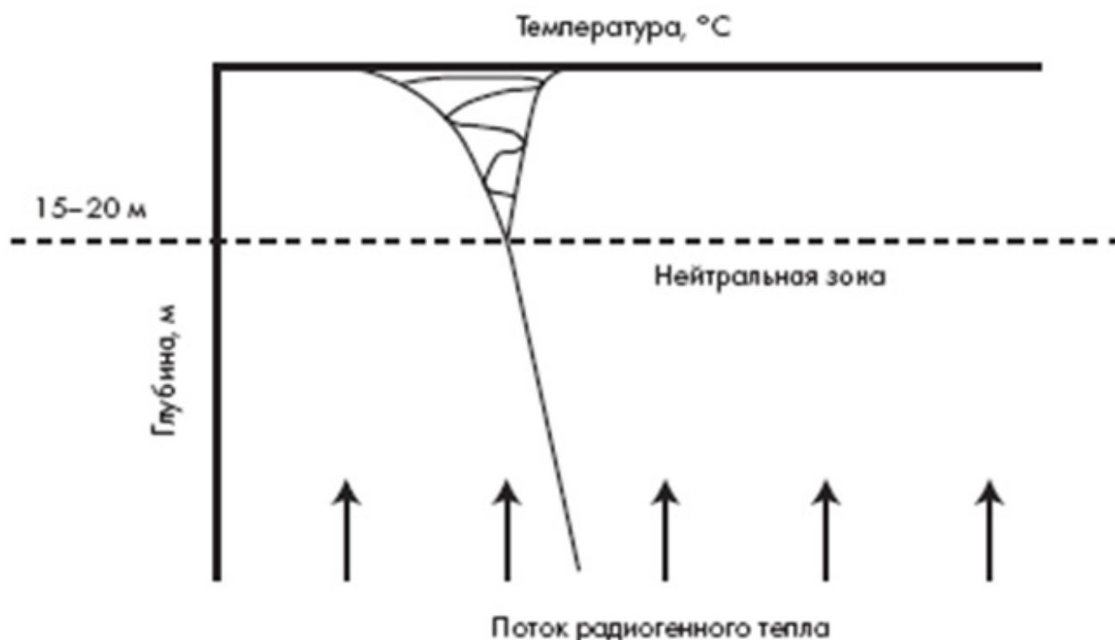
Рисунок 1 - График изменения температуры грунта в зависимости от глубины
