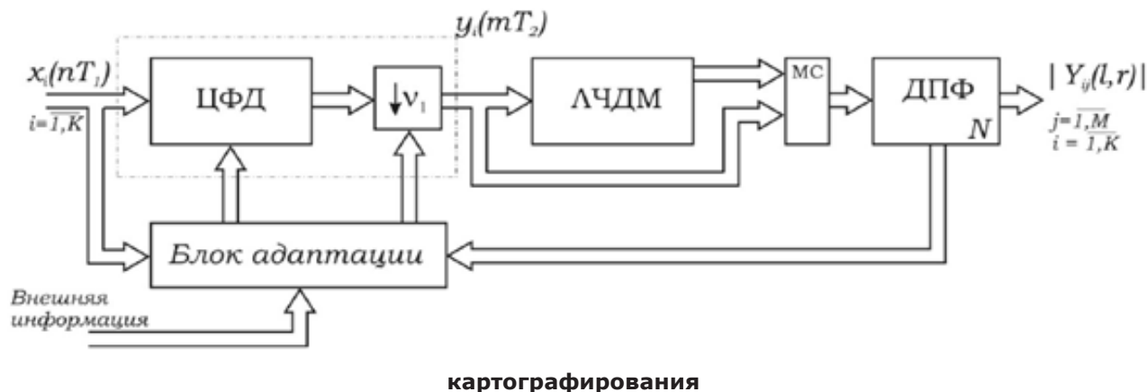
Рисунок 2-Структурная схема цифрового приемника траекторного сигнала в режимах
