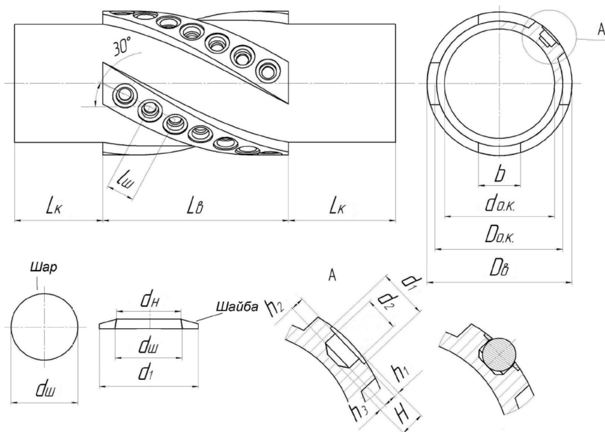
Рисунок. Центратор-турбулизатор
