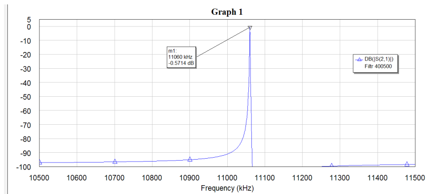
Рисунок 5 – АЧХ кварцевого фильтра в полосе 1 МГц (MWO)
