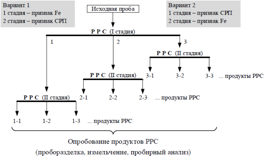
Рисунок 3 - Технологическая схема укрупненных испытаний
