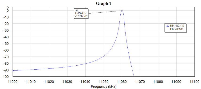
Рисунок 4 – АЧХ кварцевого фильтра в полосе 100 кГц (MWO)
