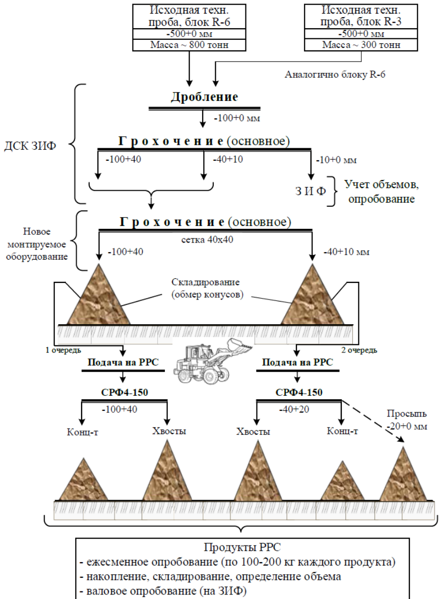
Рисунок 4 – Общая технологическая схема
