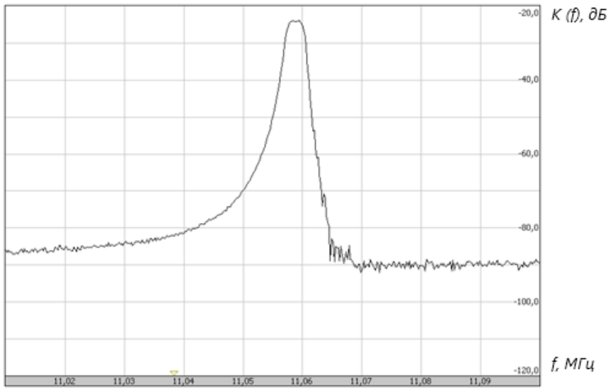
Рисунок 7 - АЧХ кварцевого фильтра в полосе 100 кГц
