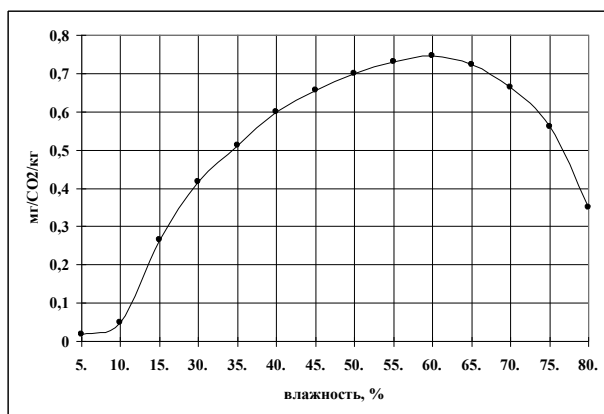
Рис. 3. Влияние влажности на интенсивность микробного дыхания почвы
