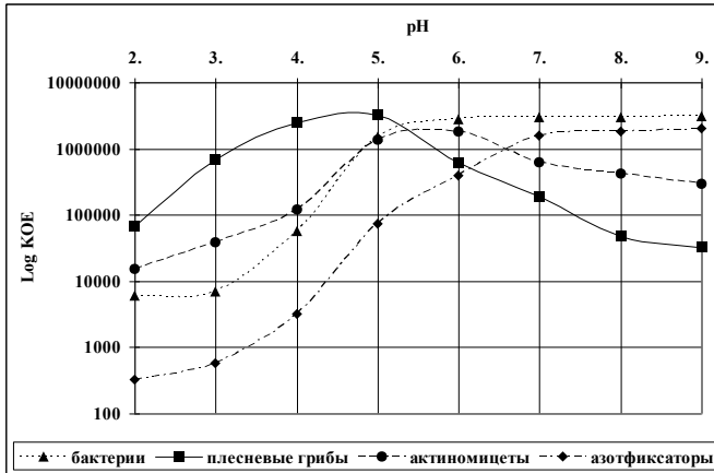
Рис. 4. Изменение численности микробной популяции в зависимости от pH почвы
