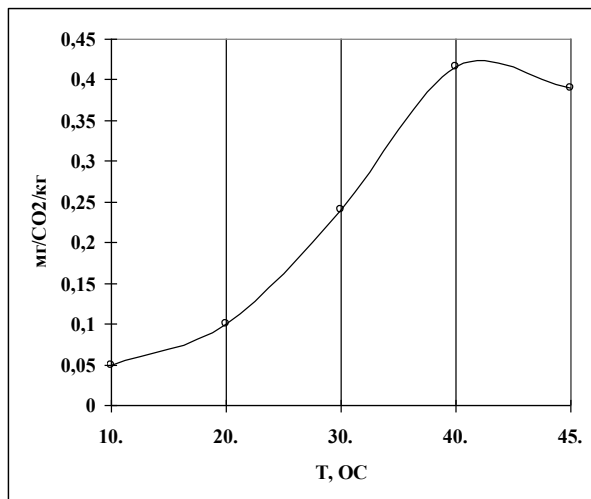
Рис. 2. Влияние температуры на интенсивность микробного дыхания почвы
