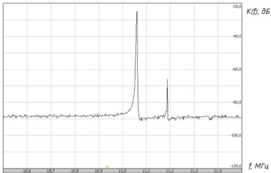
Рисунок 8 - АЧХ кварцевого фильтра в полосе 1 МГц
