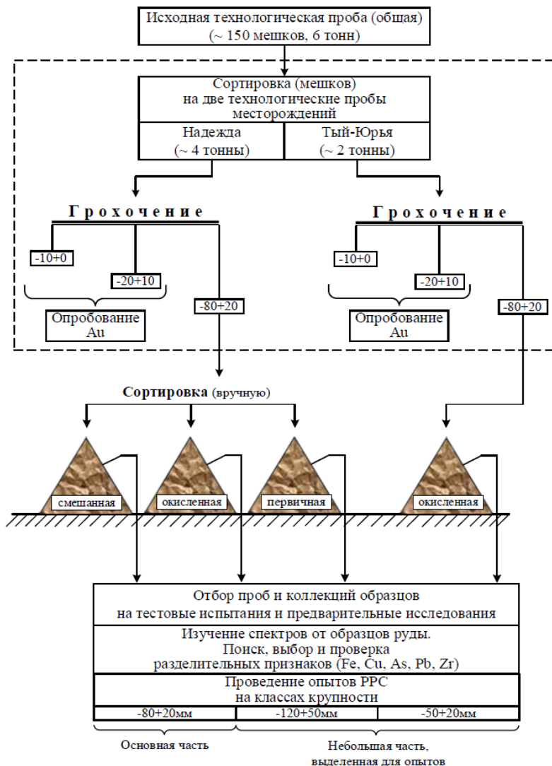
Рисунок 1 - Технологическая схема тестовых испытаний и предварительных исследований
