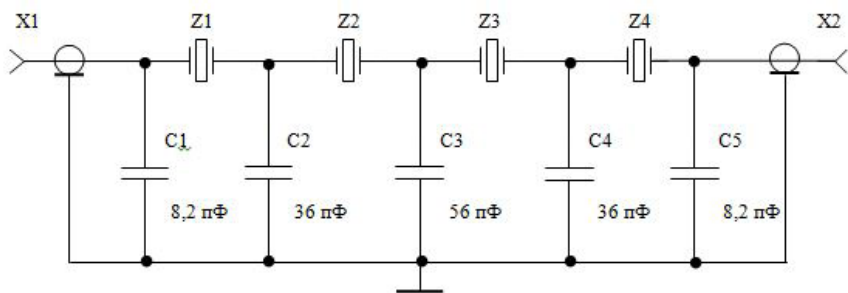
Рисунок 1 – Принципиальная схема кварцевого фильтра
