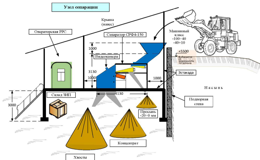
Рисунок 5 - Опытно-промышленная установка РРС (ОПУ РРС)
