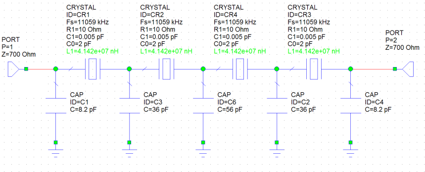
Рисунок 3 – Модель кварцевого фильтра в MWO
