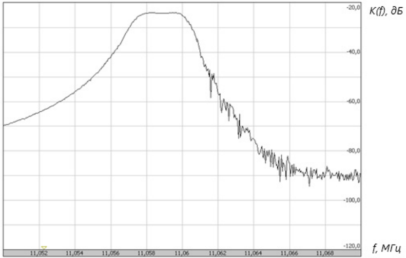
Рисунок 6 - АЧХ кварцевого фильтра в полосе 20 кГц
