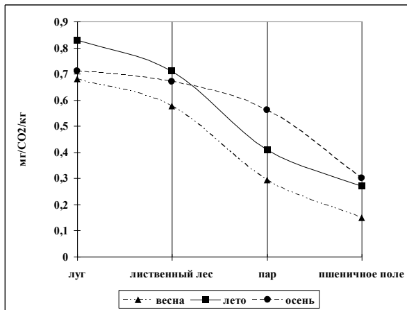
Рис. 1. Эмиссия углекислого газа с поверхности почвы в различные сезоны года
