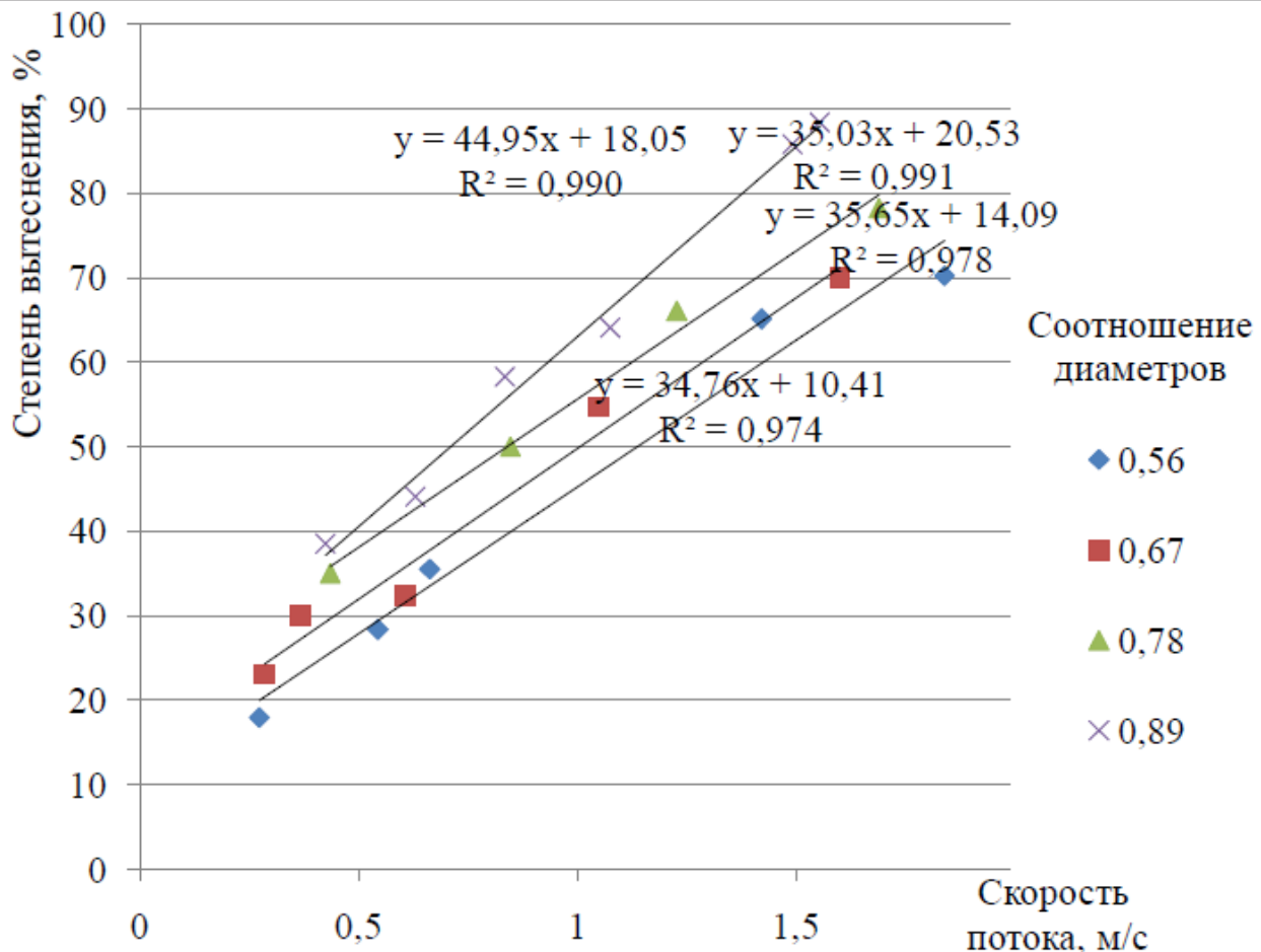
Рисунок 1. Влияние скорости потока жидкости на степень вытеснения в зависимости от соотношения d/D
