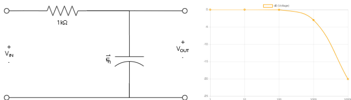
Рисунок 4. Схема и АЧХ ФНЧ.
