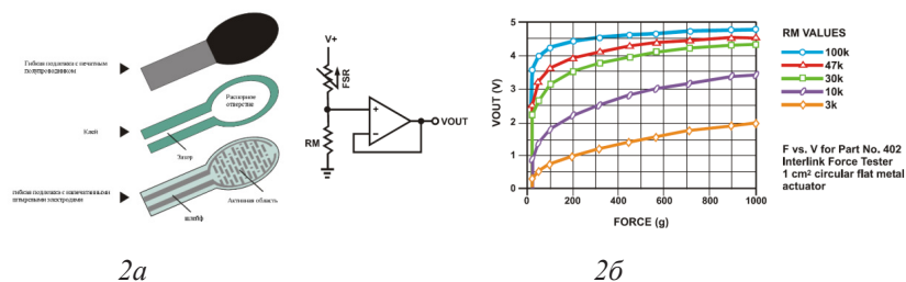
Рисунок 3. Устройство и характеристика датчика FSR402.
