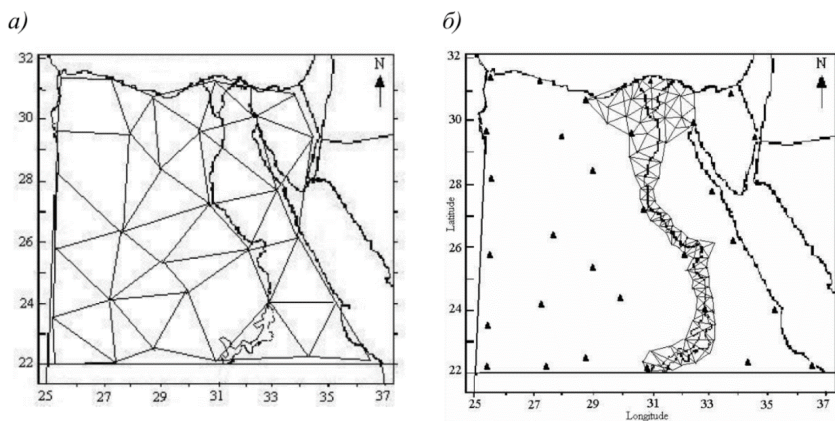
Рисунок 1. Государственная геодезическая сеть Египта.
