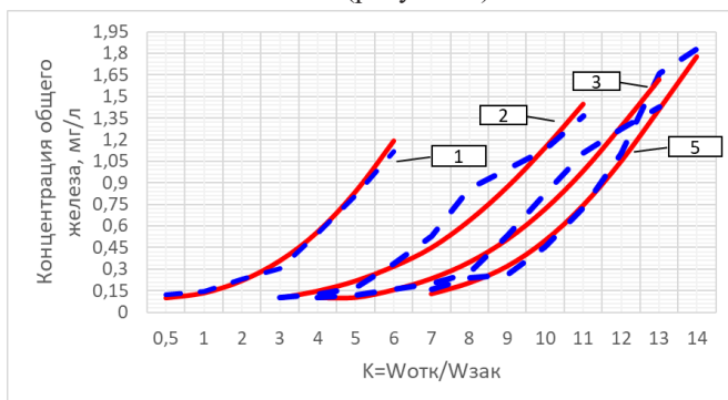
Рисунок 1. Зависимость продолжительности откачки воды в сеть с разными ее объемами закачки в подземный пласт. теоретические расчеты; экспериментальные данные; 1,2,3,5 – циклы экспериментов
