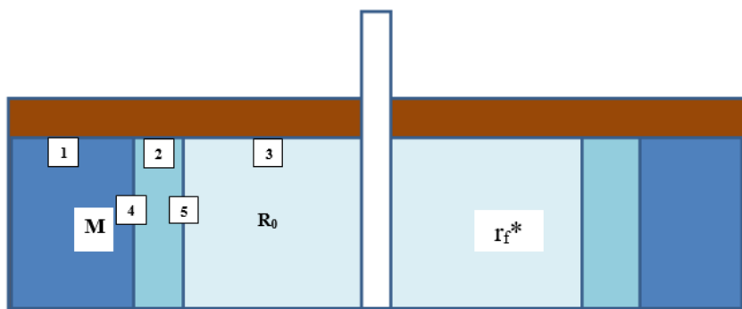
Рисунок 2. Окислительная зона вокруг скважины для определения математической модели внутрипластовой обработки воды.
