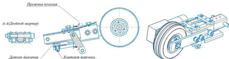
Рисунок 2. Конструкция рычага ведущего колеса.
