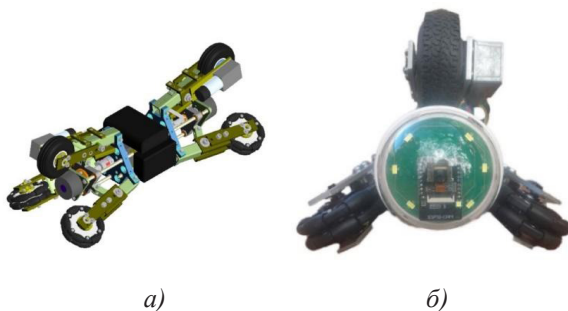
Рисунок 1. Робот для внутритрубной инспекции: а) твердотельная 3d-модель; б) прототип .
