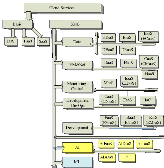
Рисунок 1. Схема классификации облачных сервисов
