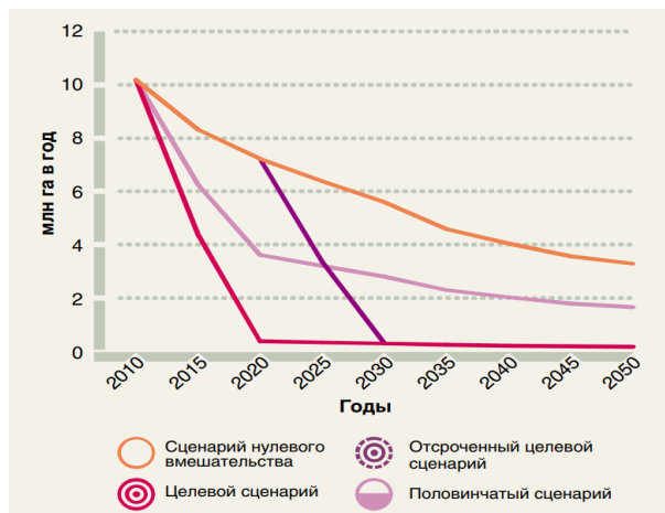
Рисунок 1. Уровни обезлесения с 2010 по 2050 год в рамках сценария нулевого вмешательства, целевого, отсроченного целевого и половинчатого сценариев
