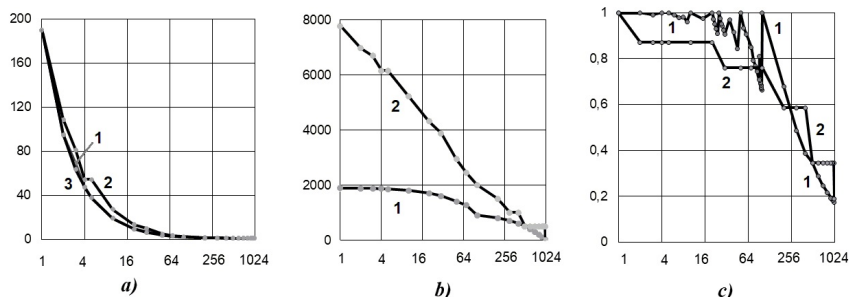
Рисунок 1. Программа t_matr_10.set (построенный по ней алгоритм) умножения квадратных матриц 10 порядка классическим методом, оси абсцисс – ширина ЯПФ после ее преобразования (фактически число отдельных машинных команд в сверхдлинном лове):
