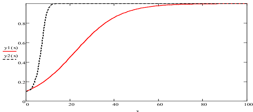
Рисунок 4. Графики роста результирующей функции по (5) y1 и (7) y2 при y = U/U_0 ; x = q ; U_0 = 1 ; U(0) = 0,1 ; \alpha = 0,1 .
