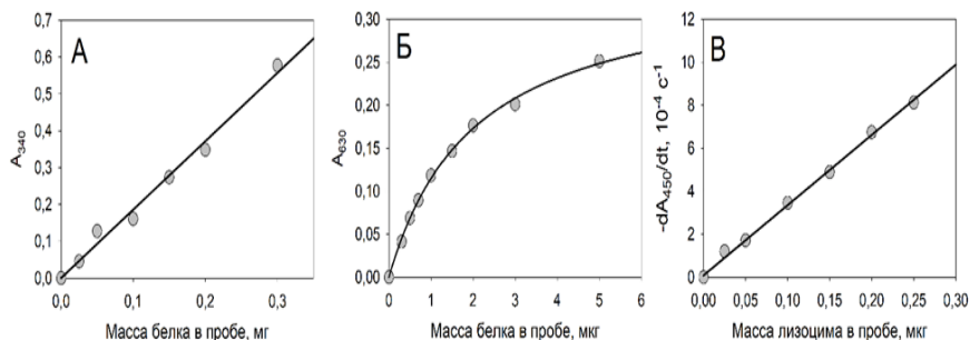
Рисунок 1. Калибровочные зависимости аналитического сигнала от массы белка-стандарта в пробе для микробиуретового метода (А), метода Брэдфорд (Б) и турбидиметрического определения активного лизоцима (В).
