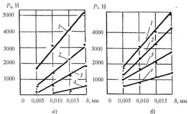
Рисунок 1. Влияние натяга и амплитуды УЗК на силы запрессовки при сборке:
