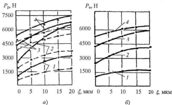
Рисунок 2. Влияние натяга и амплитуды ультразвуковых колебаний на прочность прессовых соединений (втулка и вал из стали ШХ15СГ):
